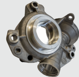
Schneckengetriebegehäuse
